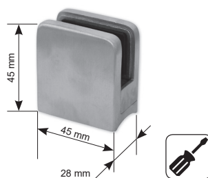
RE4743 □ 40,0x2,0 mm-es zártszelvényhez
