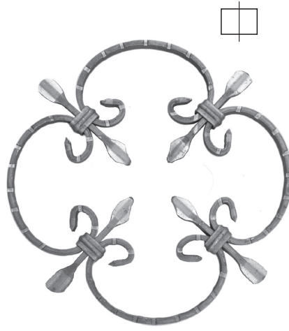
R 23/1 ▧ 10×5 mm Ø 250 mm
