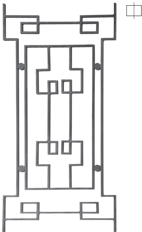
RGD 202/1 ▧ 14×8 mm 1000×500 mm
