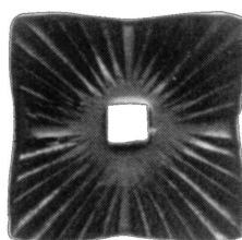
R 116/A/2 □ 75×75 mm ▽ 5 mm
