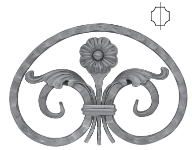
R 458/1 ▧ 14×14 mm 300×210 mm
