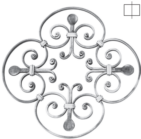
R 1655/1 □ 12×6 mm Ø 430 mm
