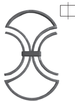
RGD 187/2 □ 14×8 mm 190×325 mm
