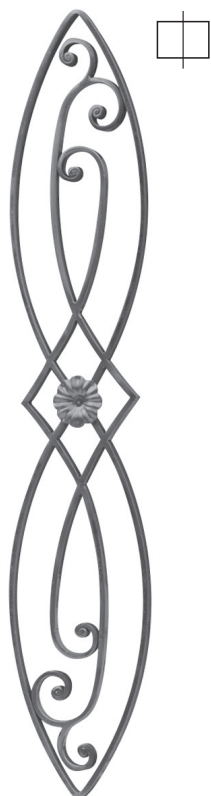
R 1681/1 □ 14×8 mm 190×1000 mm
