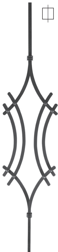
RGD 21/3 □ 12×12 mm 200×1000 mm
