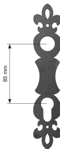
RF 9335 40×205×2 mm
