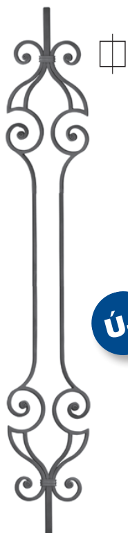
RGD 150/2 □ 14×14 mm H 1000×205 mm
