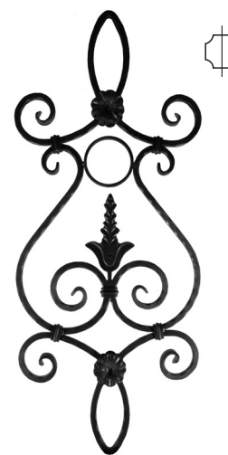
R 475/2 □ 12×12 mm 380×900 mm
