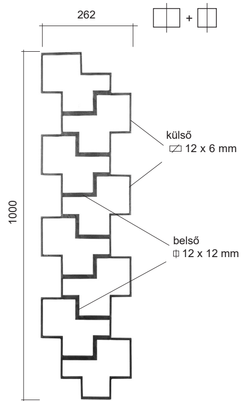
RGD 293/1 □ 12×6 mm + □ 12 mm 1000×262 mm
