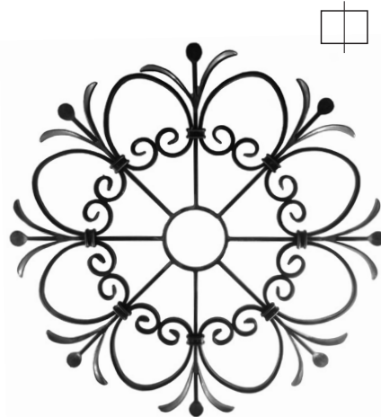
R 1020/1 □ 12×6 mm ∅ 590 mm
