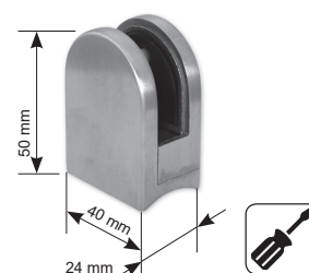
RE4760/304 □ 40,0x2,0 mm-es zártszelvényhez
