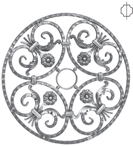
R 459/1 □ 14×14 mm Ø 610 mm
