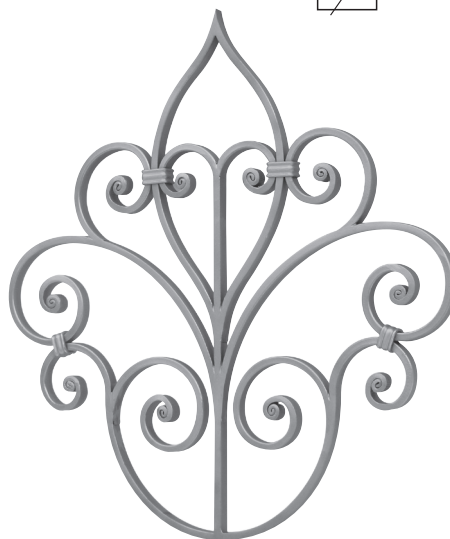
RGD 234/2 □ 14×8 mm 500 x 520 mm
