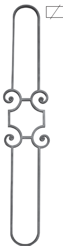
RGD 245/3 ▤ 14×8 mm 180×1000 mm
