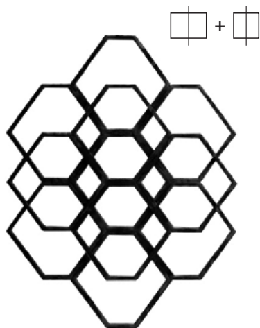
RGD 299/4 □ 16×8 mm + □ 8 mm 458×600 mm
