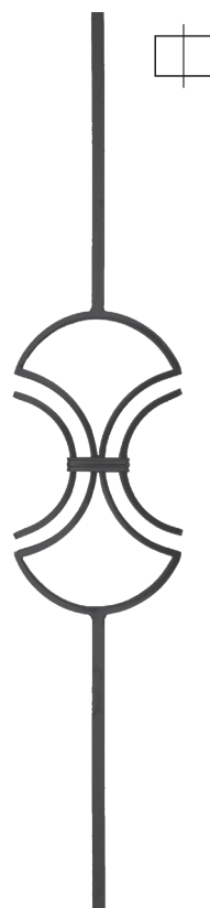
RF 9077 □ 14×8 mm H 190×1000 mm
