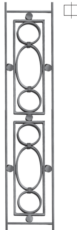
RGD 205/2 ▧ 14×8 mm 210×1000 mm
