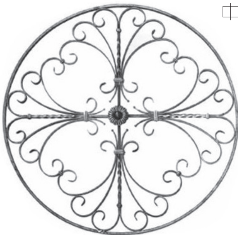
R 457/2 □ 12×6 mm Ø 1045 mm
