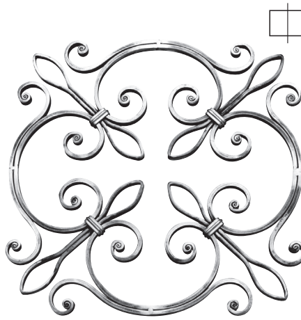
R 1667/2 □ 14×8 mm Ø 470 mm
