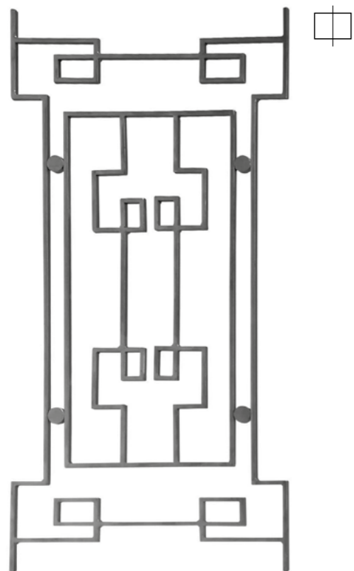
RGD 202/1 ▧ 14×8 mm 1000×500 mm
