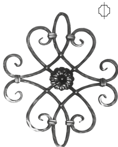
R 26/C/1 □ 12×12 mm 430×530 mm
