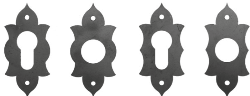
RF 9333 40×80×2 mm RF 9334 40×80×2 mm RF 9331 40×80×2 mm RF 9332 40×80×2 mm
