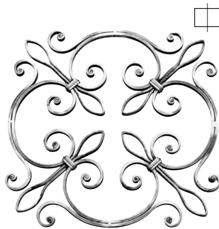
R 1667/2 □ 14×8 mm ∅ 470 mm
