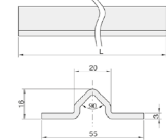
R 101.60 Ø 60 mm, szögvasra terhelés: 100 kg
