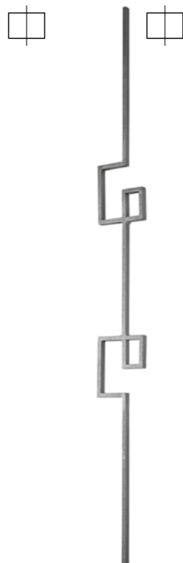
RGD 202/2 ▧ 14×8 mm 1000×95 mm
