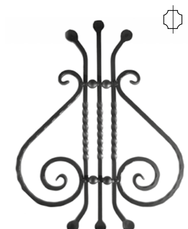
R 460/2 □ 12×12 mm 460×600 mm
