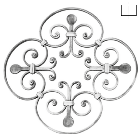
R 1655/1 □ 12×6 mm ∅ 430 mm
