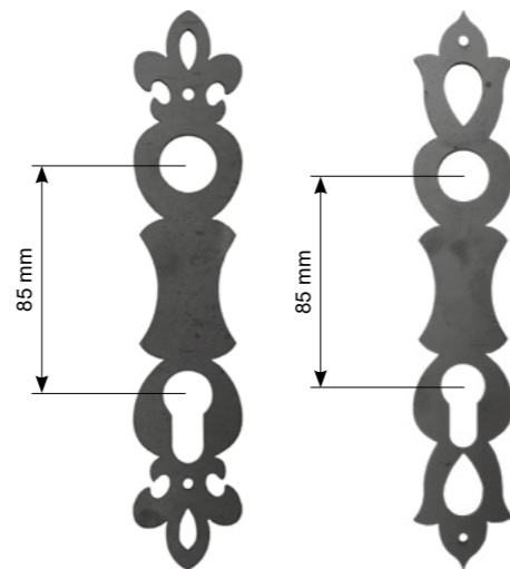
RF 9335 40×205×2 mm RF 9336 40×225×2 mm
